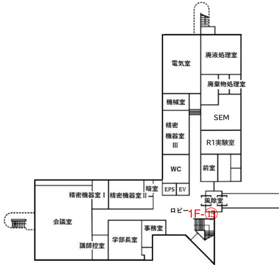
1階 平面図
