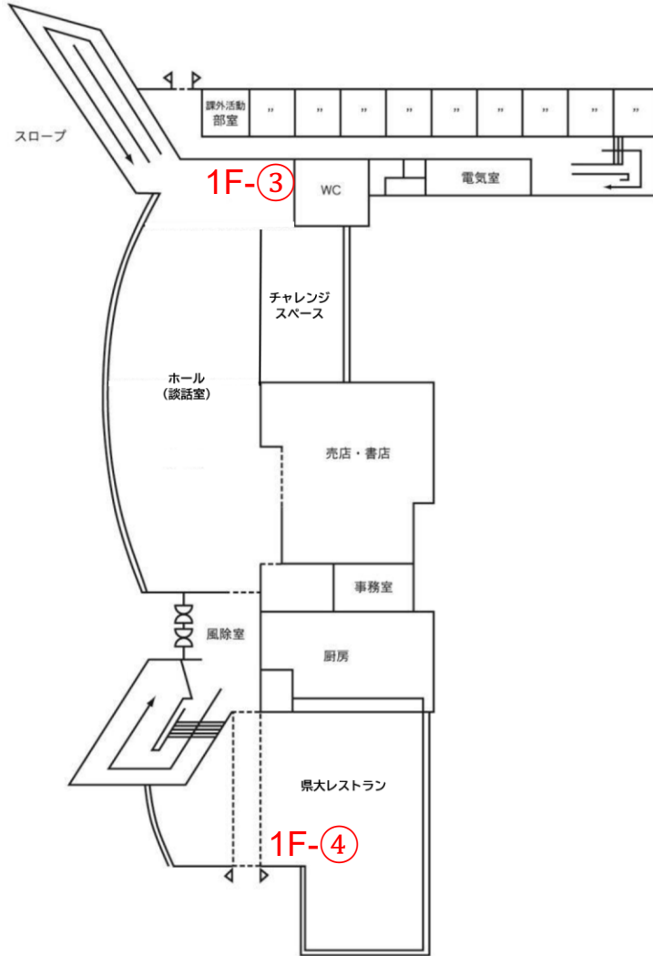
1階 平面図
