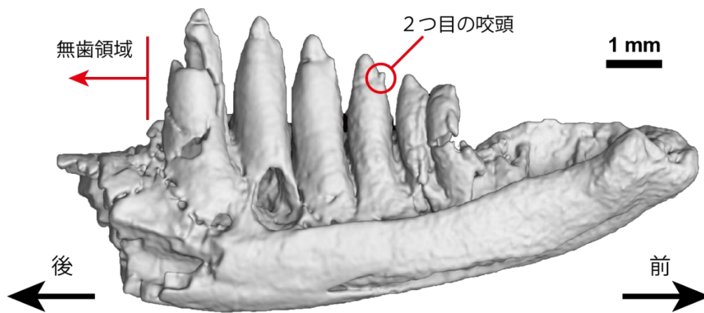
勝浦町のトカゲ類化石の特徴（内側から見た図）
