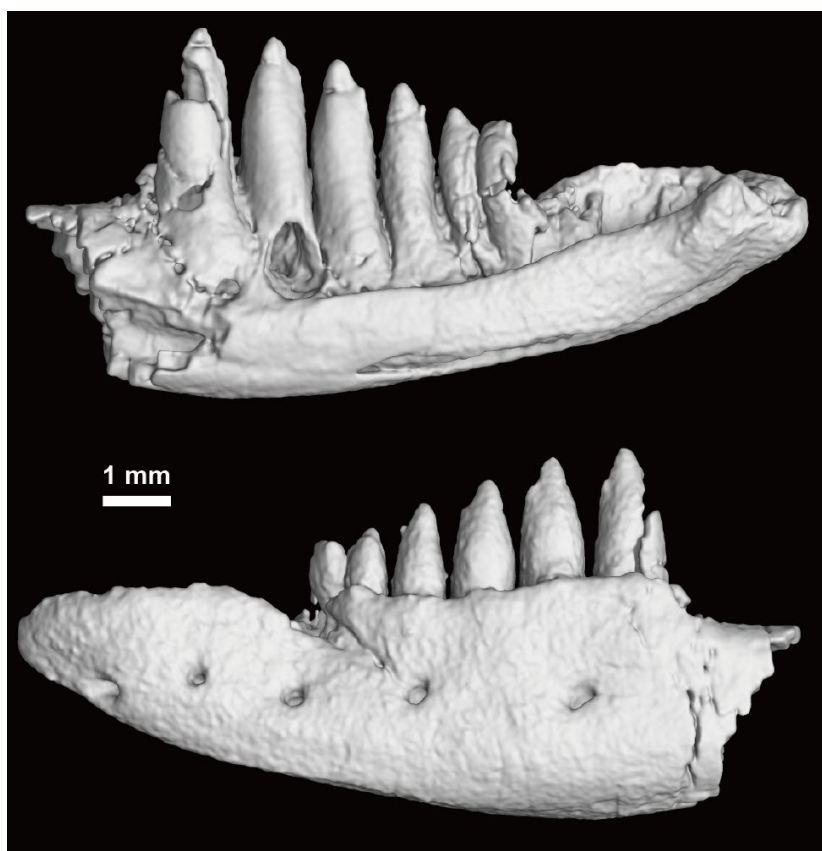
3次元再構築モデル（上：内側、下：外側）
