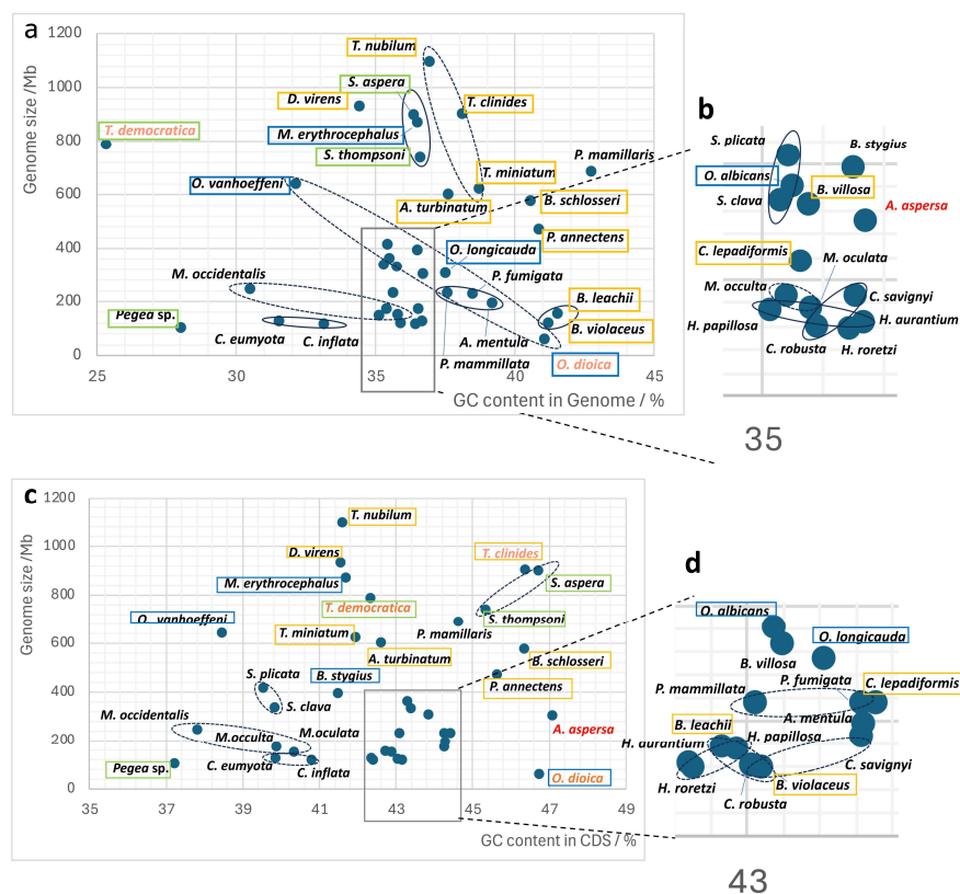
図 2 : ゲノムサイズと GC 含量の多様性。 (a) 38 種の被囊類について、ゲノム全体の GC 含量（横軸）とゲノムサイズ（縦軸）をプロットしたもの。(b) (a) の密集部分の拡大図。(c) 遺伝子のコード領域（CDS）の GC 含量とゲノムサイズの関係。(d) (c) の密集部分の拡大図。被囊類のゲノムサイズは約 17 倍、GC 含量も 25.3～42.7%と大きく異なる。 A. aspersa (赤字) は、コード領域の GC 含量が 38 種のなかで最も高い (47.1%) という際立った特徴をもつ。種名は各系統の分類・生活様式に応じて色分けした四角形で示す。囲いなし：単体・固着（ホヤ綱）、黄枠：群体・固着（ホヤ綱）、青枠：単体・浮遊（オタマボヤ綱）、緑枠：群体・浮遊（タリヤ綱）。
